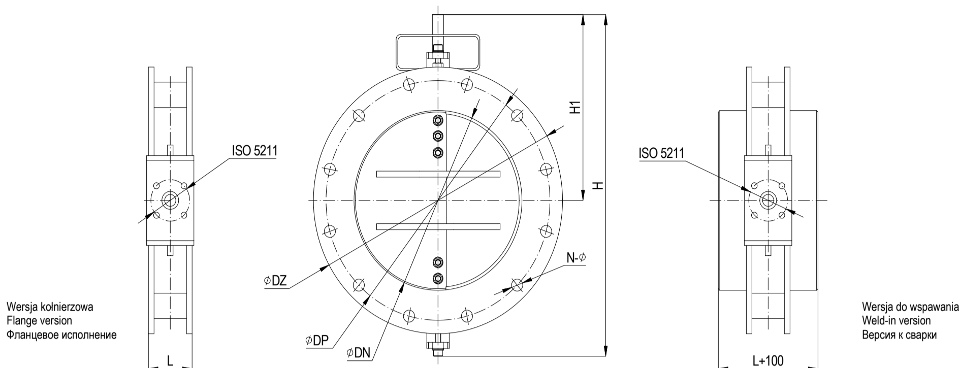
Rys. 1. Główne wymiary urządzenia w wersji krótkiej | Main dimensions of the device in short version | Основные размеры устройства в короткой версии
