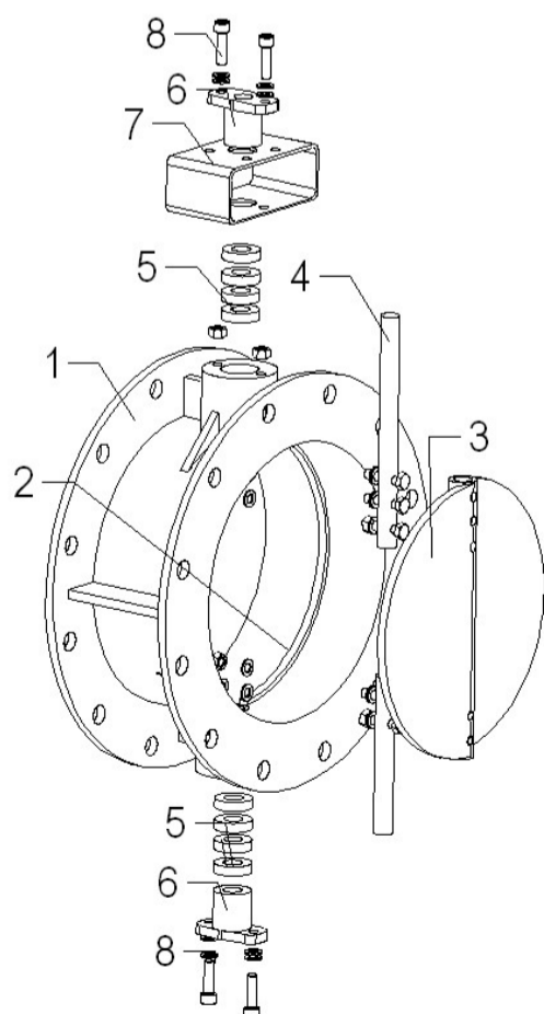
Rys. 2. Rysunek złożeniowy | Exploded view | В разобранном виде
