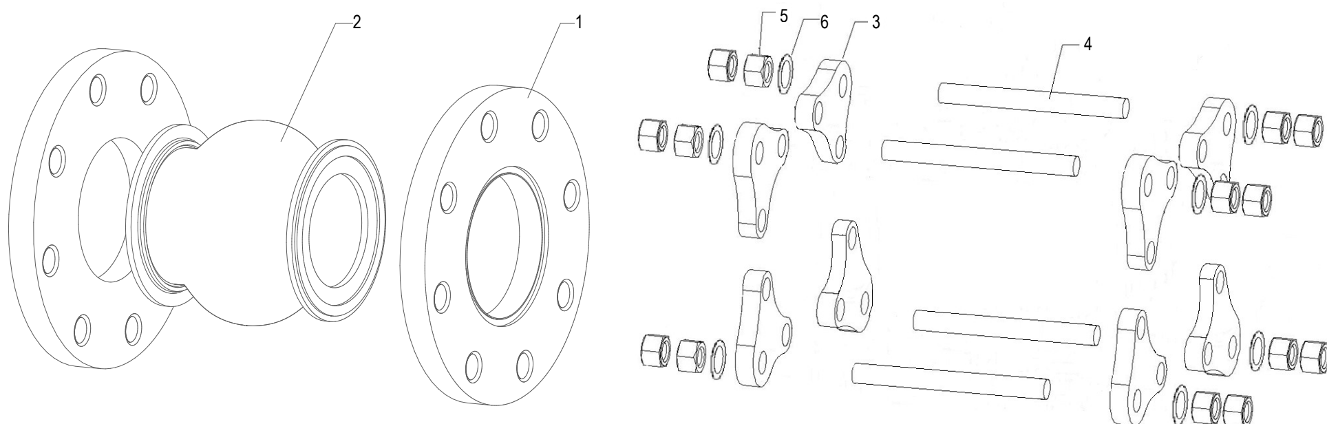
Rys. 2. Rysunek złożeniowy | Exploded view | В разобранном виде
